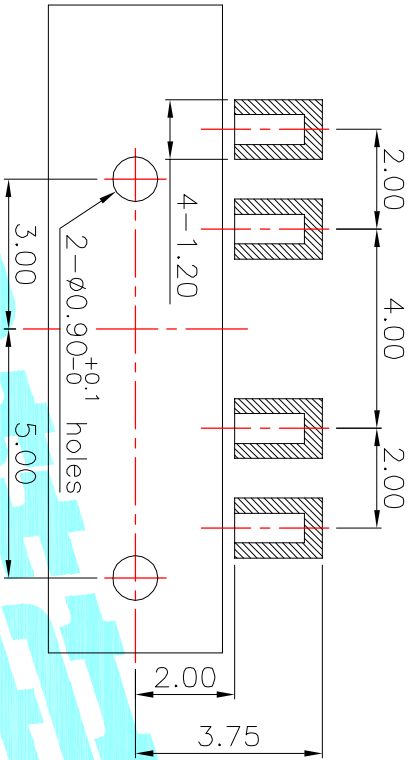
PCB Layout(Pattern side)
